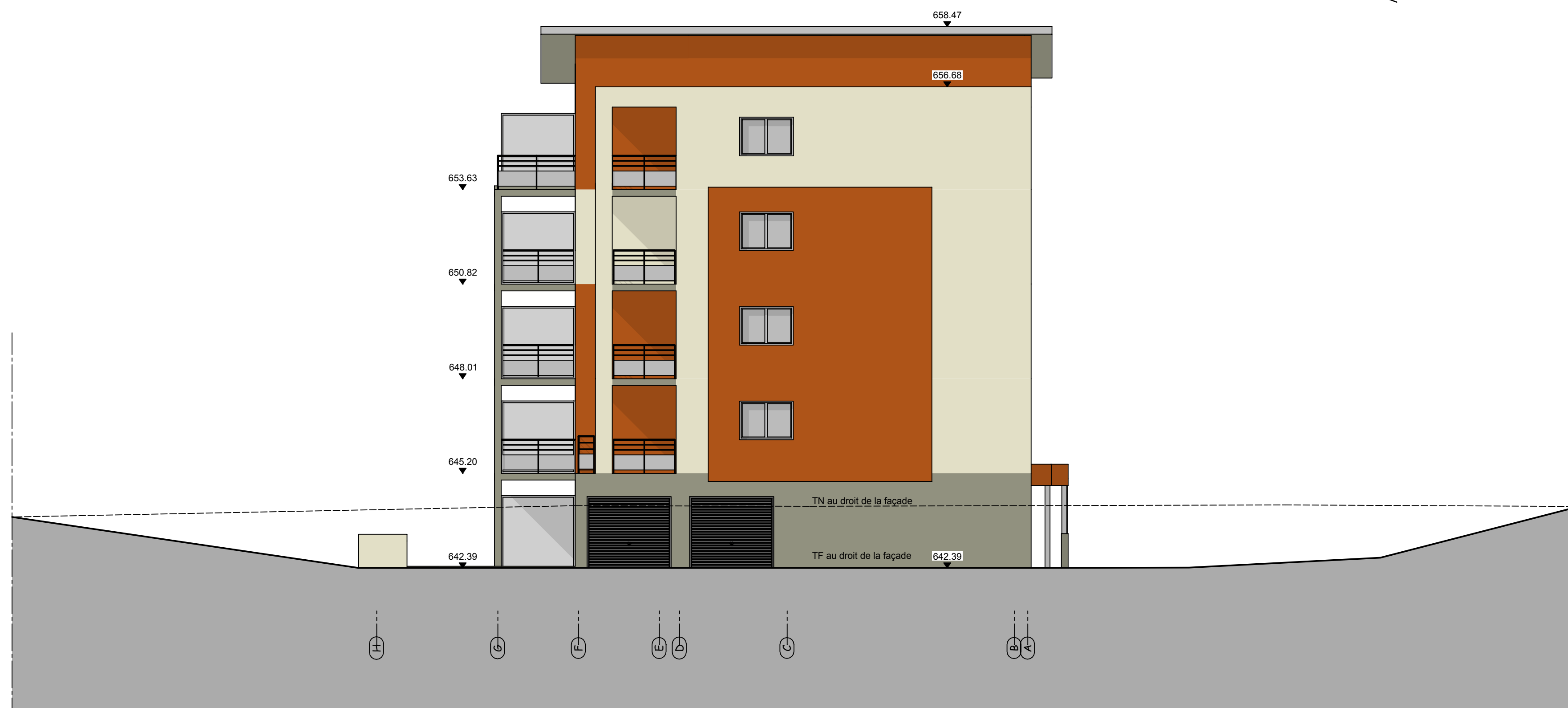
FACADE NORD-EST
